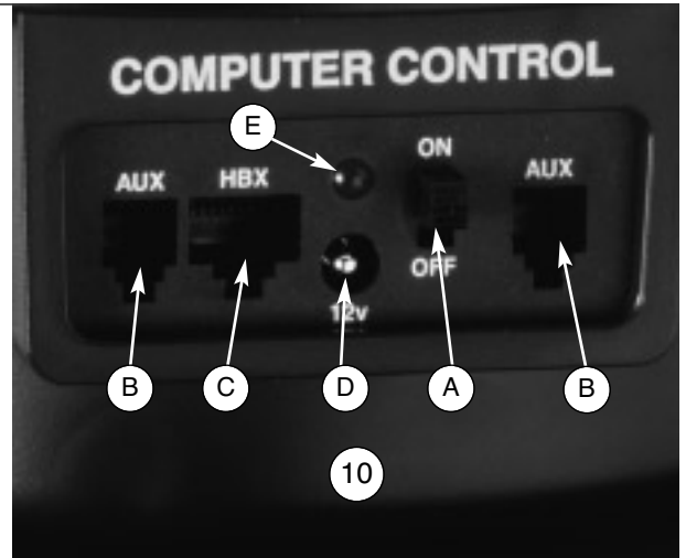
Fig 2 : Panneau de contrôle. (A) interrupteur d'alimentation "ON/OFF" (marche/arrêt) ; (B) ports auxiliaires ; (C) port de la raquette de commande ; (D) prise 12 V ; (E) diode lumineuse clignotante indicatrice de mise sous tension
