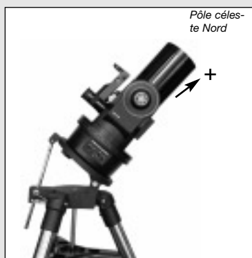
Fig. 49 : exemple d'alignement polaire. Notez que l'avant du plateau incliné fait face au Nord. C'est la position de départ.
