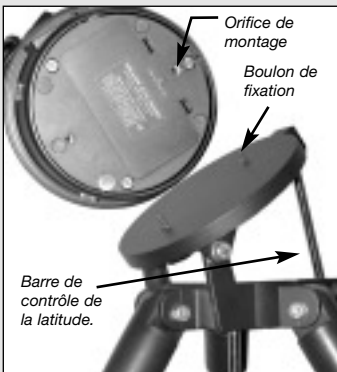
Fig. 45 : orifice de montage de la jambe haute de latitude et boulon de fixation correspondant.
