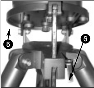
Fig. 10 : desserrage du levier
