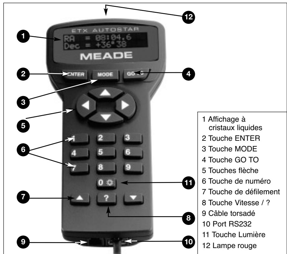
Fig. 4 : Raquette de commande Autostar
