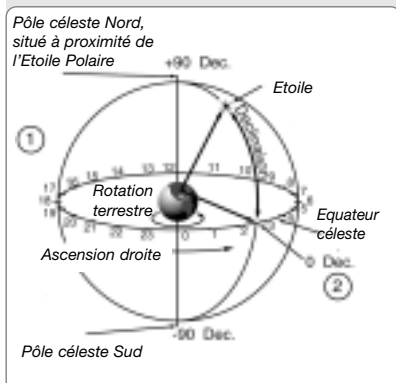
Fig. 43 : sphère céleste
