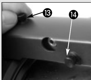
Fig. 18 : Tournez les vis de réglage du Smartfinder du dessus (13) ou du côté (14).
